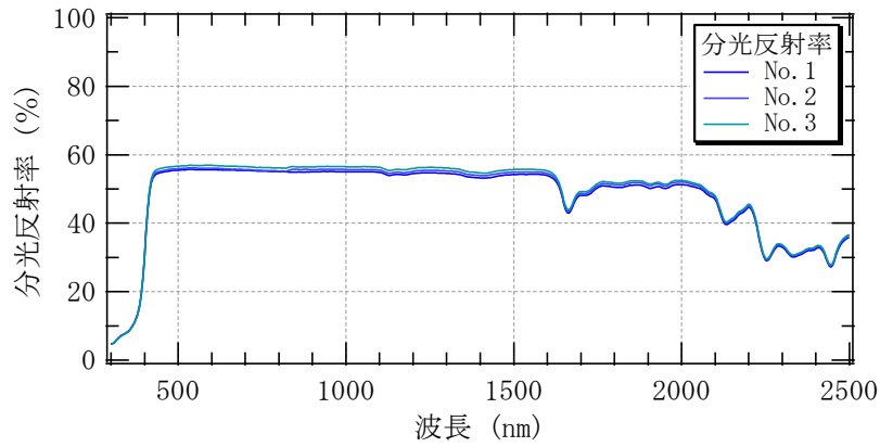
図 5-4 分光反射率測定結果（色番号 6345）
