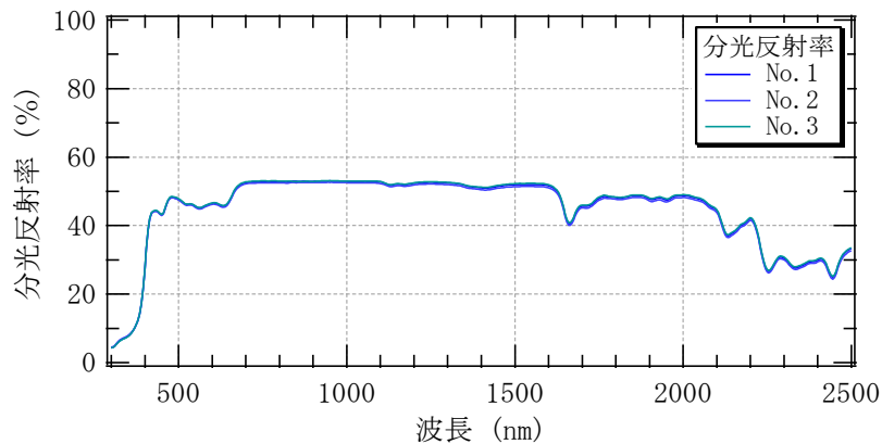
図 5-6 分光反射率測定結果（色番号 6347）
