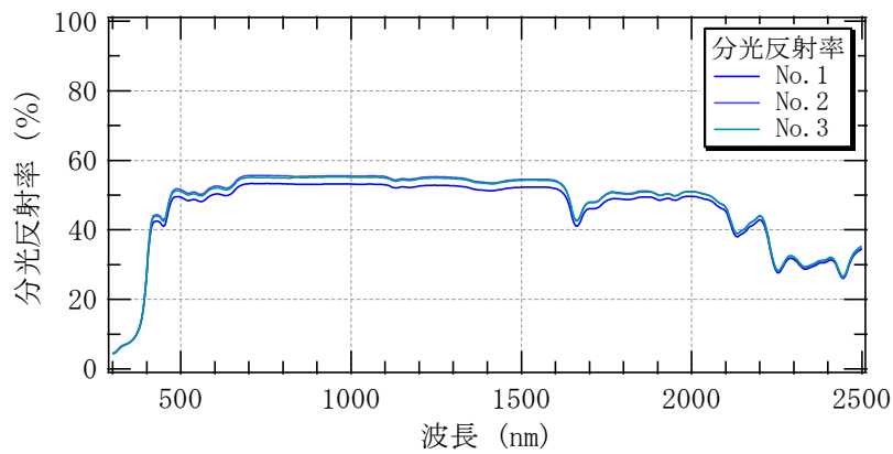
図 5-5 分光反射率測定結果（色番号 6346）
