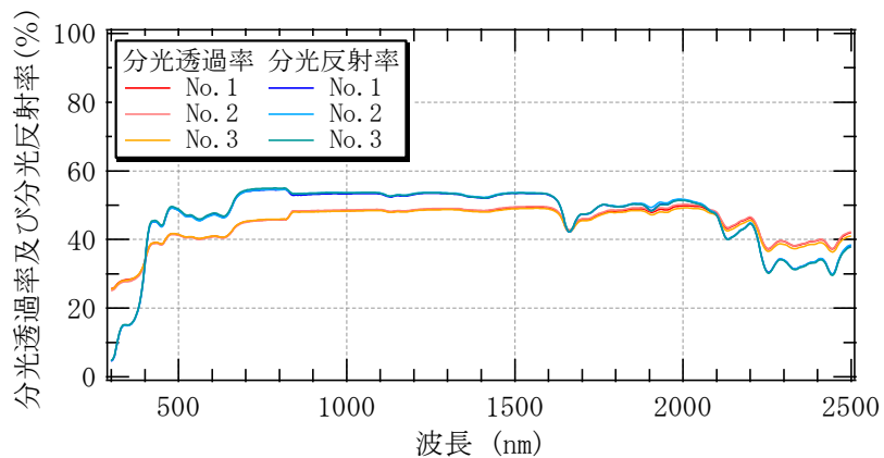
図 5-3 分光透過率及び分光反射率測定結果（色番号 6347）
