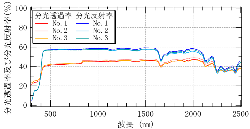
図 5-1 分光透過率及び分光反射率測定結果（色番号 6345）
