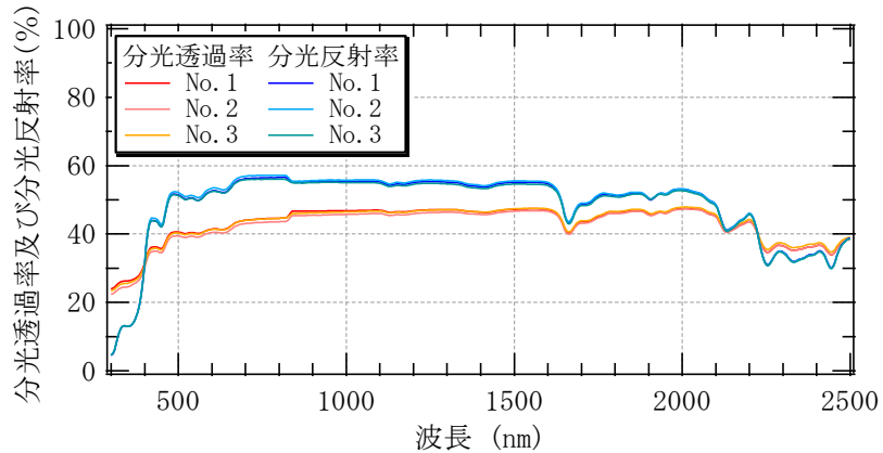
図 5-2 分光透過率及び分光反射率測定結果（色番号 6346）
