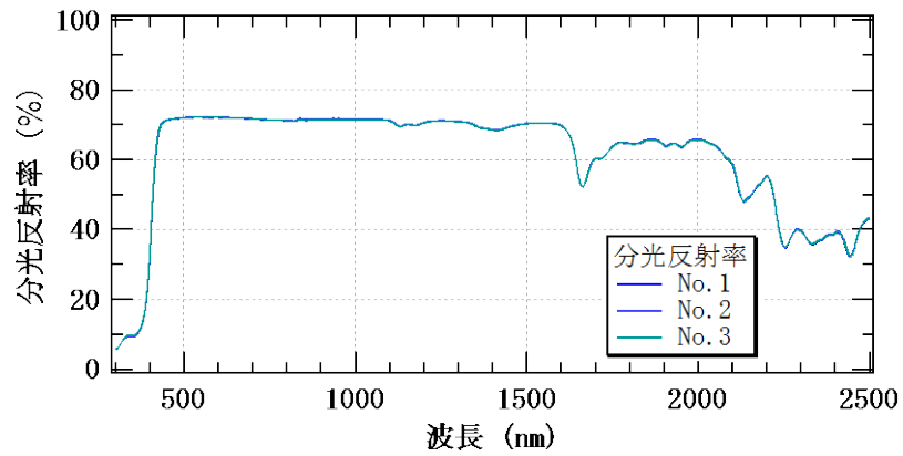
図 5-4 分光反射率測定結果（色番号 6297）
