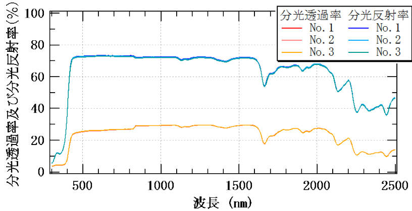
図 5-1 分光透過率及び分光反射率測定結果（色番号 6297）
