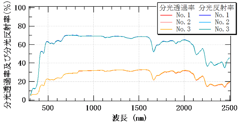
図 5-2 分光透過率及び分光反射率測定結果（色番号 6298）
