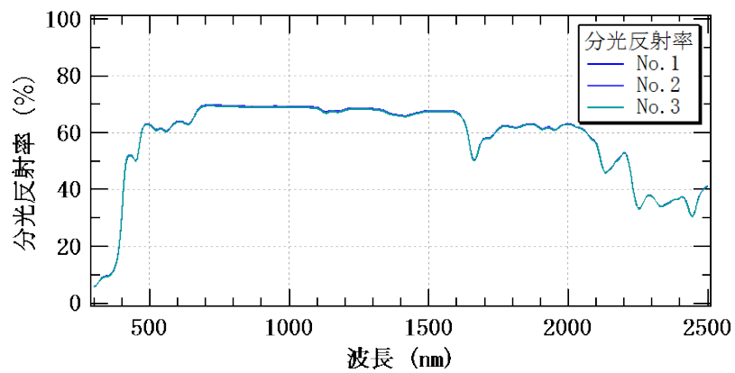
図 5-5 分光反射率測定結果（色番号 6298）
