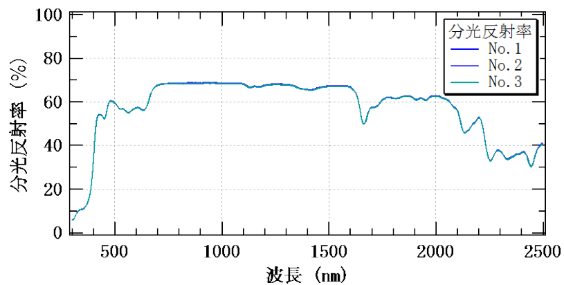
図 5-6 分光反射率測定結果（色番号 6298）
