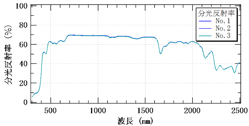
図-5 分光反射率測定結果（色番号 6298）
