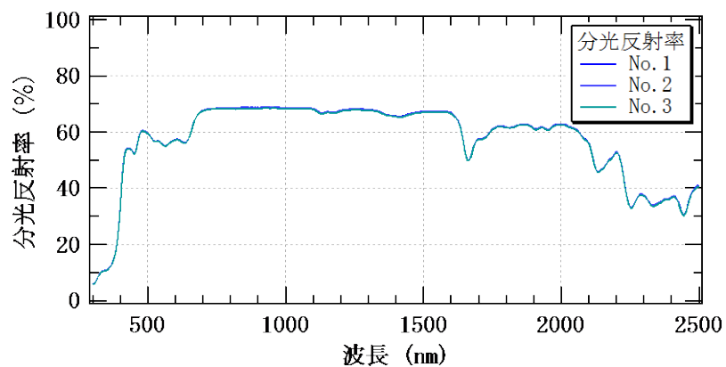
図-6 分光反射率測定結果（色番号 6299）
