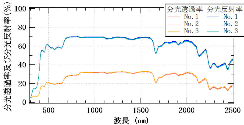
図 5-3 分光透過率及び分光反射率測定結果（色番号 6299）
