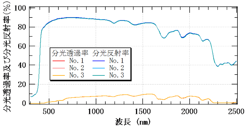
図 5-2 分光透過率及び分光反射率測定結果（色番号 6270）
