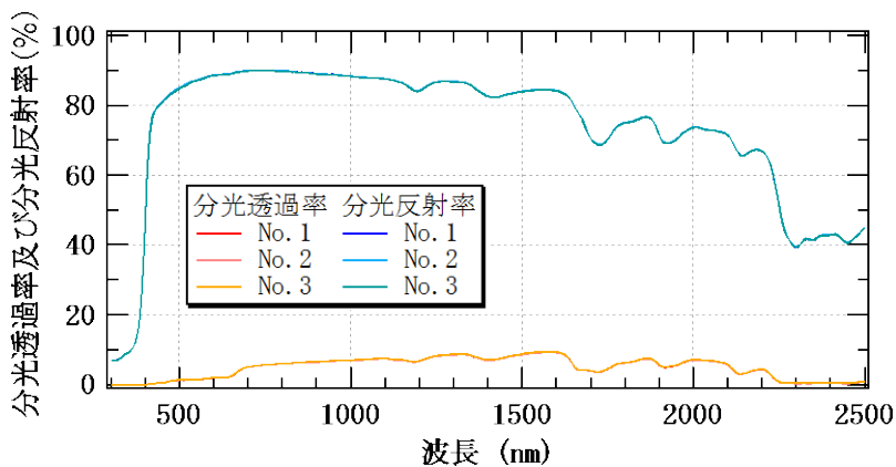
図 5-3 分光透過率及び分光反射率測定結果（色番号 6271）
