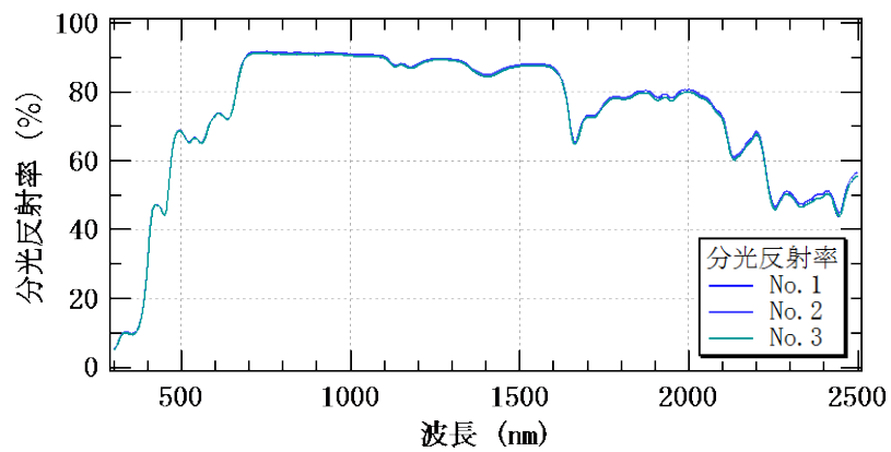
図 5-5 分光反射率測定結果（色番号 6270）
