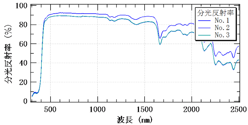
図 5-4 分光反射率測定結果（色番号 6269）
