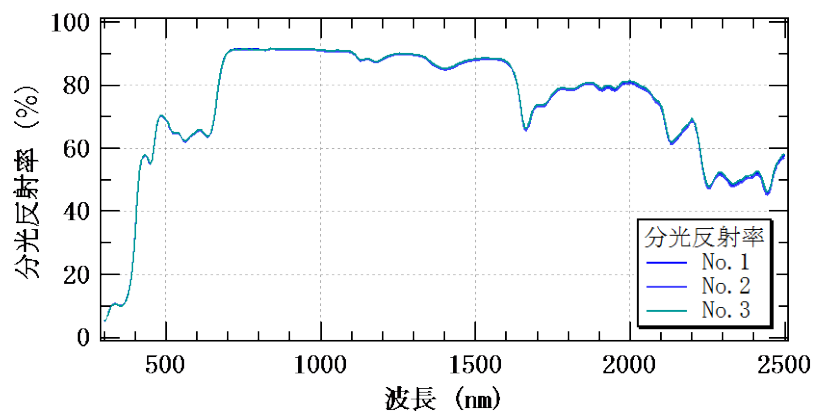
図 5-6 分光反射率測定結果（色番号 6271）
