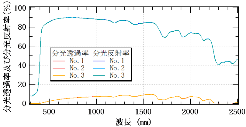
図 5-1 分光透過率及び分光反射率測定結果（色番号 6269）
