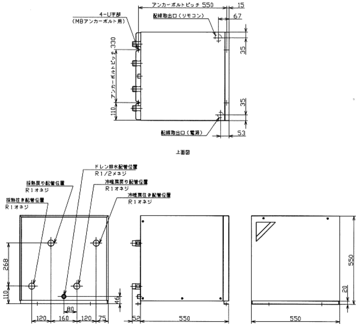
図 3-3 実証対象技術外形図（地中熱ヒートポンプユニット GSHP-1002URF）
