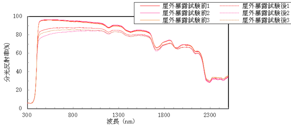
図 5-3 分光反射率測定結果（白色）
