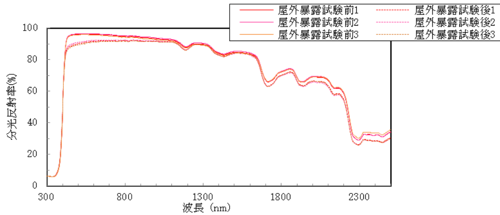
図 2 分光反射率測定結果 (白色)
