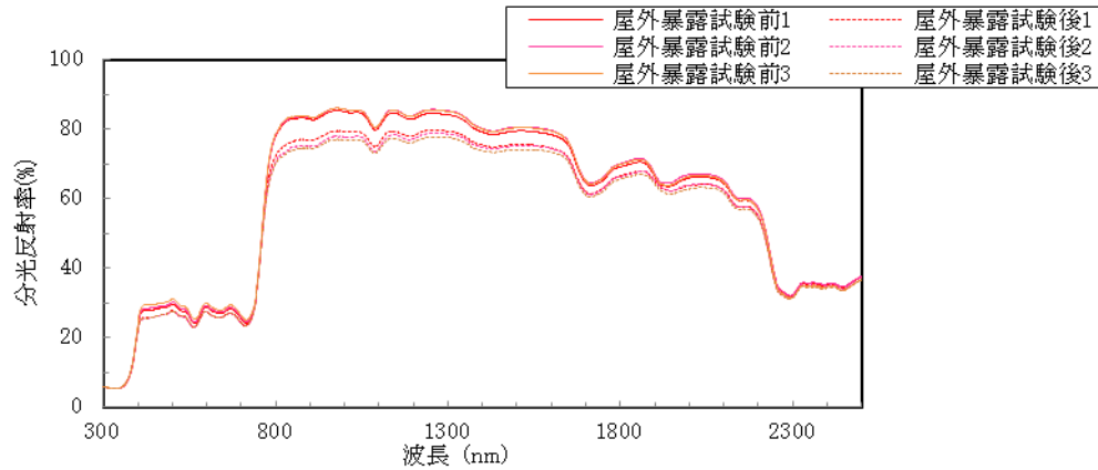
図 5-2 分光反射率測定結果（灰色）
