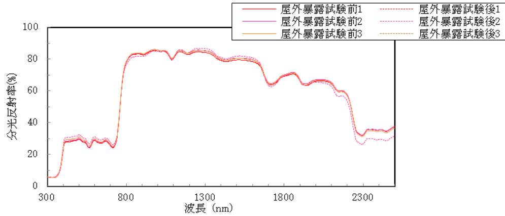
図 1 分光反射率測定結果 (灰色)
