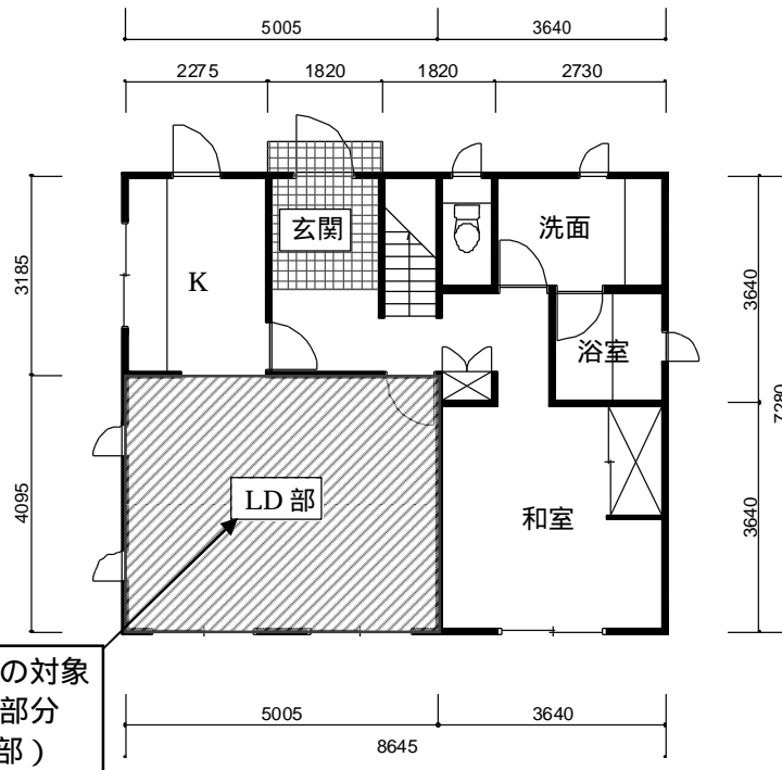
図 4-1 計算用住宅モデル (平面図)
