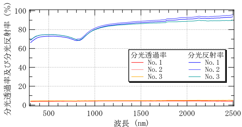
図 5-2 分光透過率及び分光反射率測定結果 (ダークグレー)
