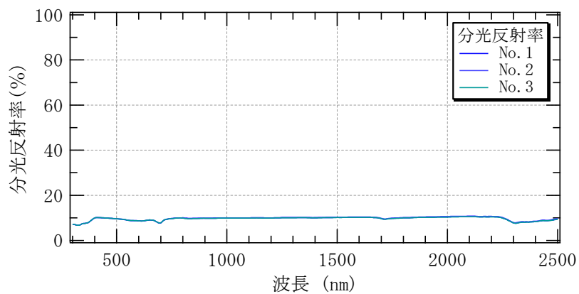
図 5-4 分光反射率測定結果 (ダークグレー)
