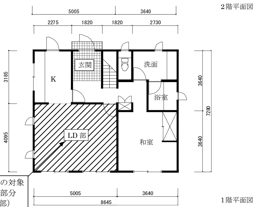
図 4-1 計算用住宅モデル (平面図)
