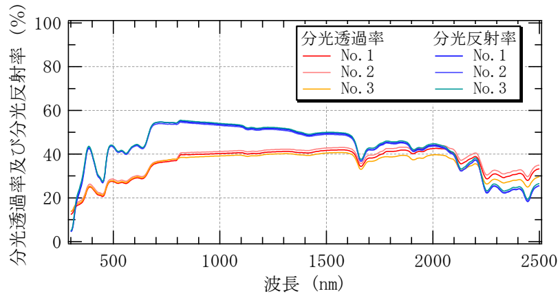
図 5-2 分光透過率及び分光反射率測定結果 (ベージュ)
