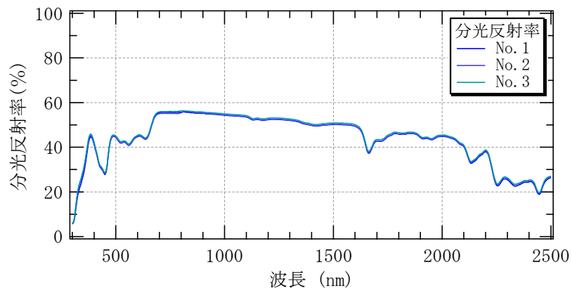
図 5-4 分光反射率測定結果 (ベージュ)
