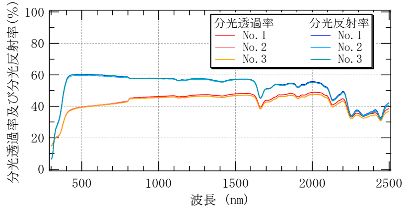
図 5-1 分光透過率及び分光反射率測定結果 (白)
