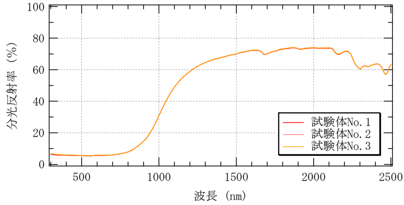
図 5-2 分光反射率測定結果 (C063S [ブラック])
