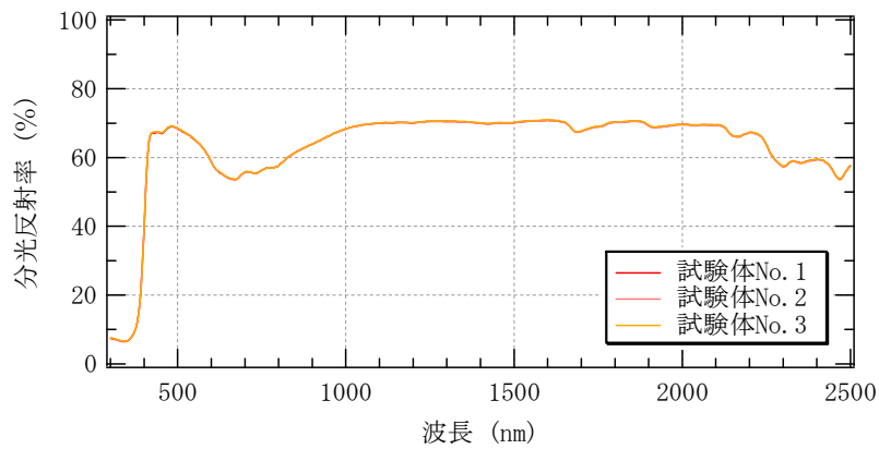
図-3 分光反射率測定結果 (C018S [パールブルー])
