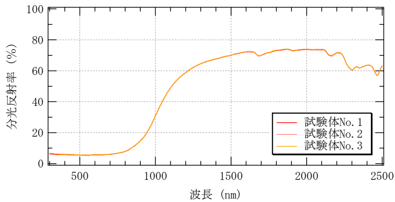
図-2 分光反射率測定結果 (C063S [ブラック])
