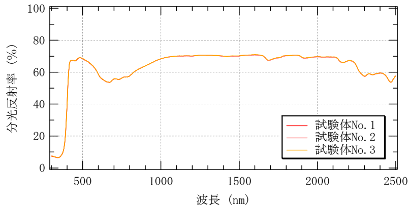
図 5-3 分光反射率測定結果 (C018S [パールブルー])
