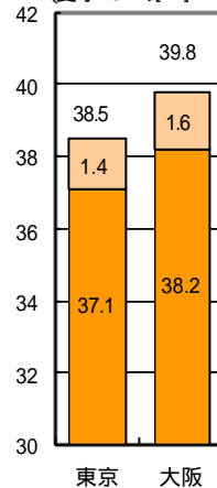
自然室温上昇抑制効果 (住宅) (夏季15時) [℃]
