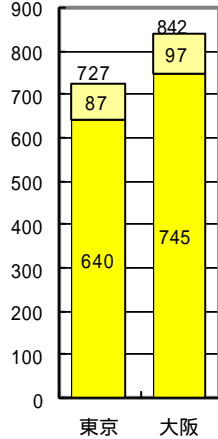
冷房負荷低減効果 (住宅) (夏季1ヶ月) [kWh]
