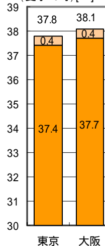
自然室温上昇抑制効果(オフィス) (夏季15時)[ ]
