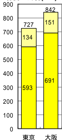
冷房負荷低減効果 (住宅)
