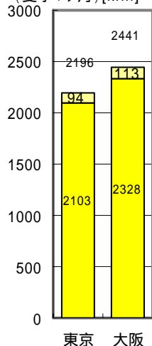
冷房負荷低減効果 (オフィス)
