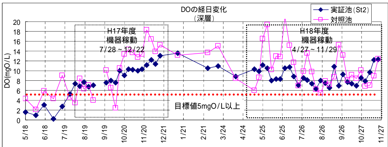
図5 - 2 DO経日変化 (深層)
