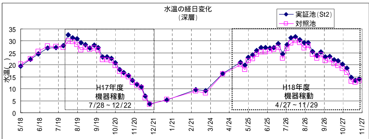
図5 - 5 水温経日変化 (深層)
