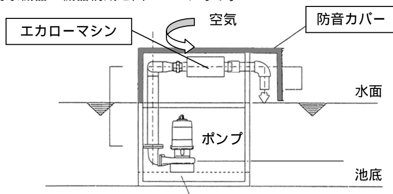
図2 - 1 実証対象機器（エカローシステム）の機器構成
