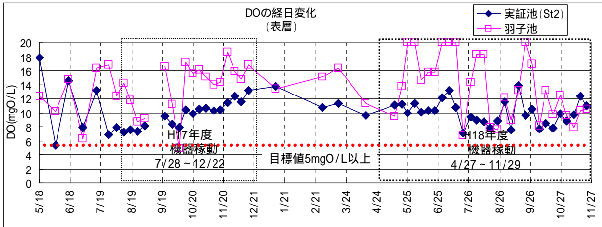
図5 - 1 DO経日変化 (表層)
