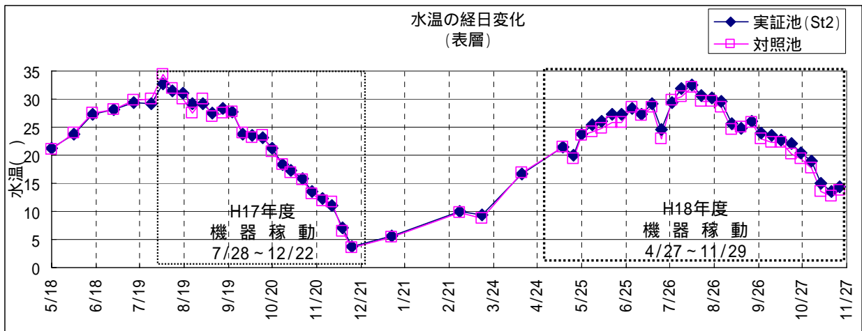
図5 - 4 水温経日変化 (表層)
