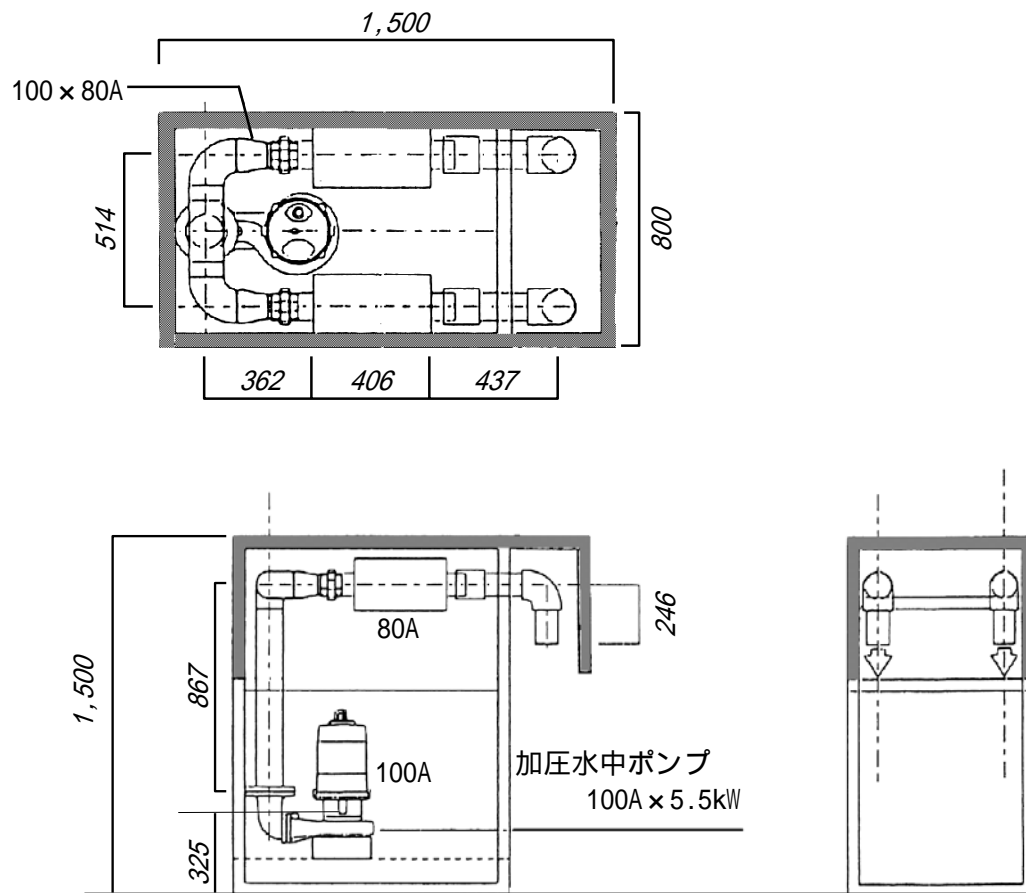
図 2 - 2 実証対象機器（エカローシステム）本体の三面図
