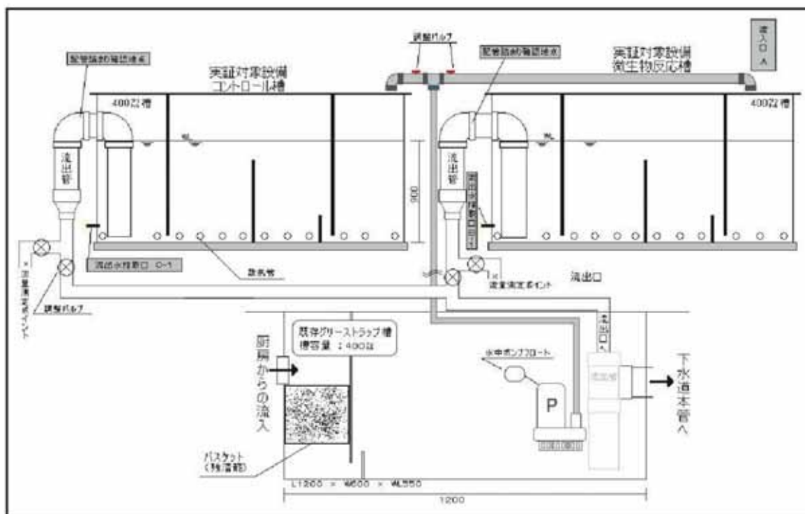
図 2 - 2 処理フロー
