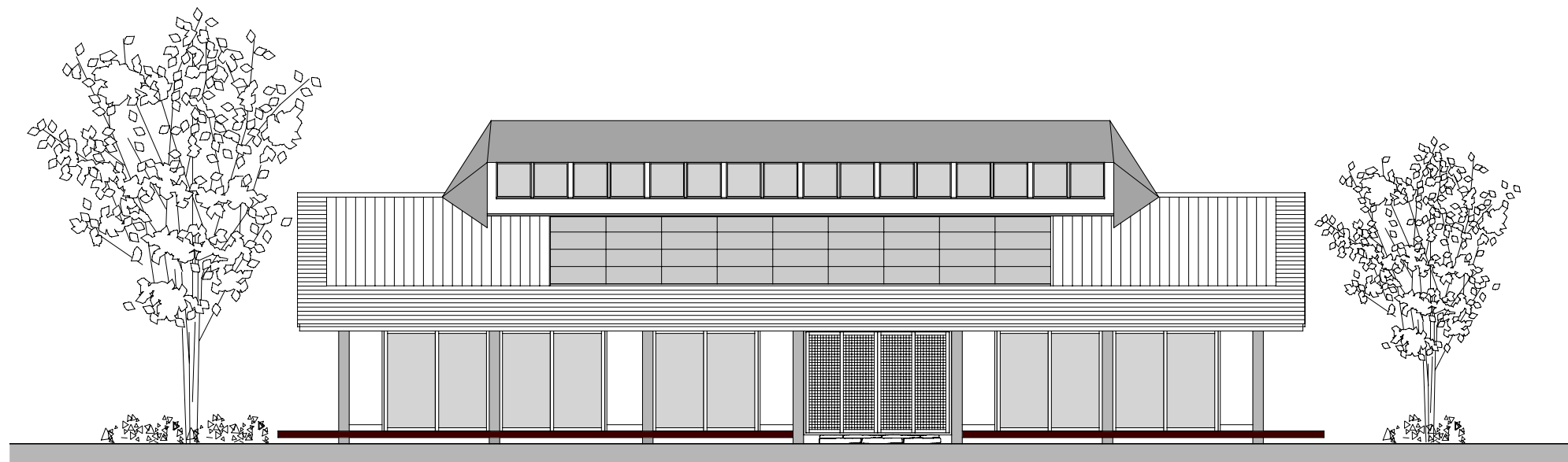
南立面図 1/100
