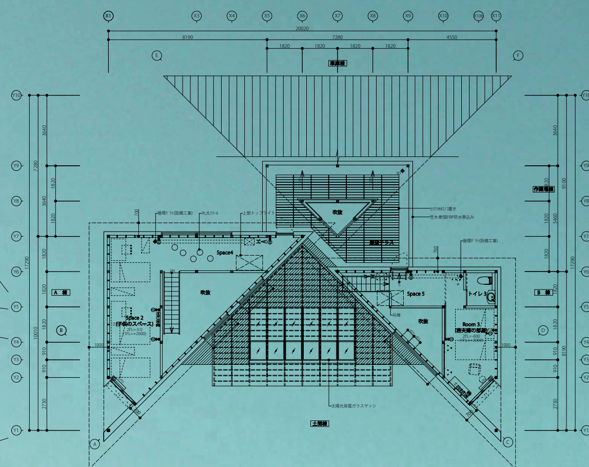
2階平面図 1/200
