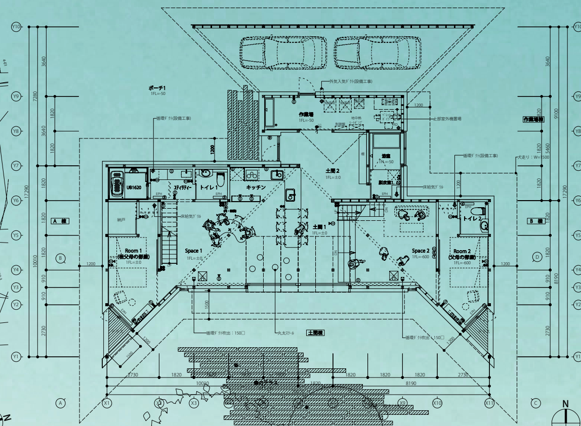
1階平面図 1/200
