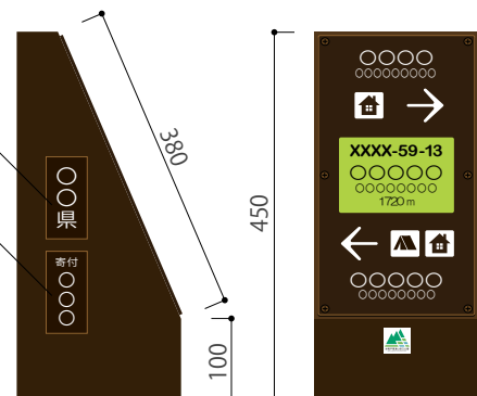
側面
