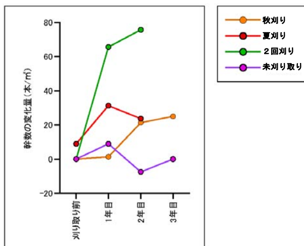
図 3-8 稈数の推移
