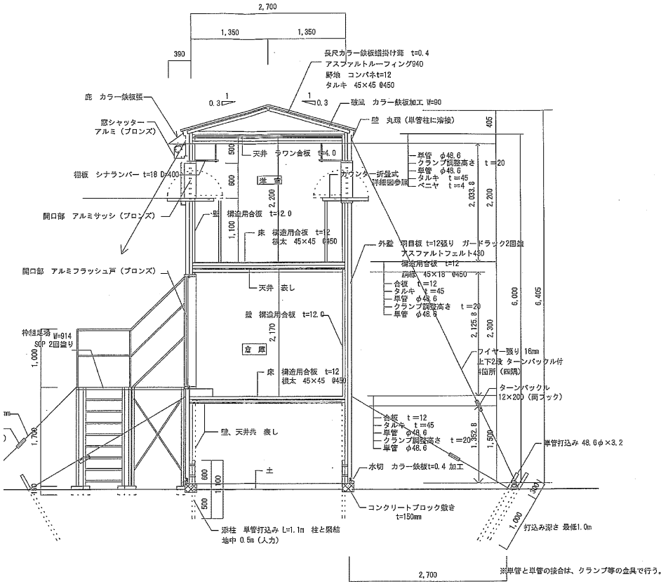
ハイシート断面図 S=1/100
