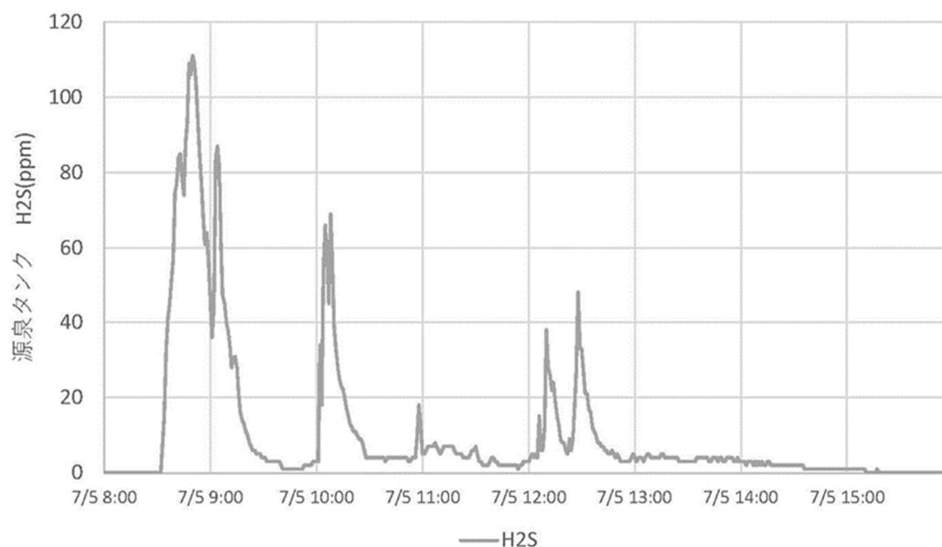
図1 アルカリ性硫黄泉（pH8.8）の貯湯槽内空気中硫化水素濃度の変化 （間欠湯沸しており、ポンプ稼働すると濃度が上昇する）
