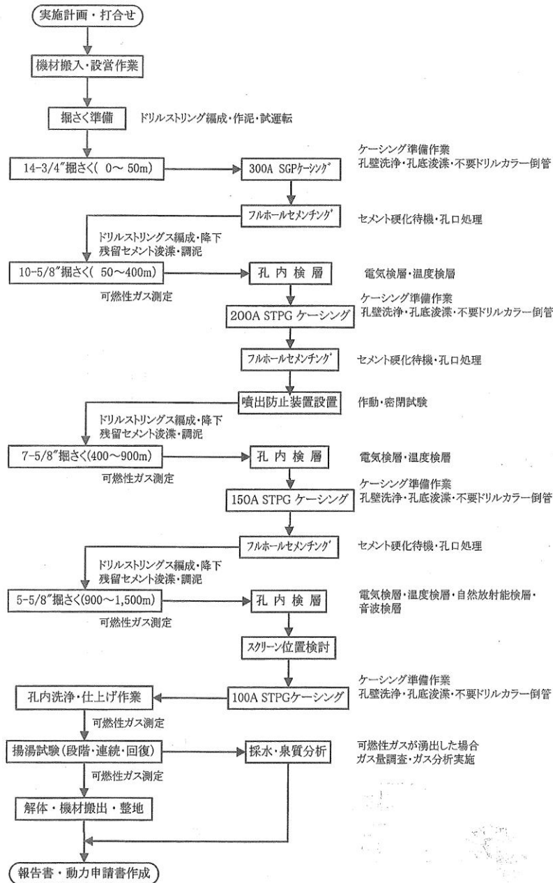
図 1.3.1 温泉掘さく作業手順図 (掘さく深度 1,500mの例)
