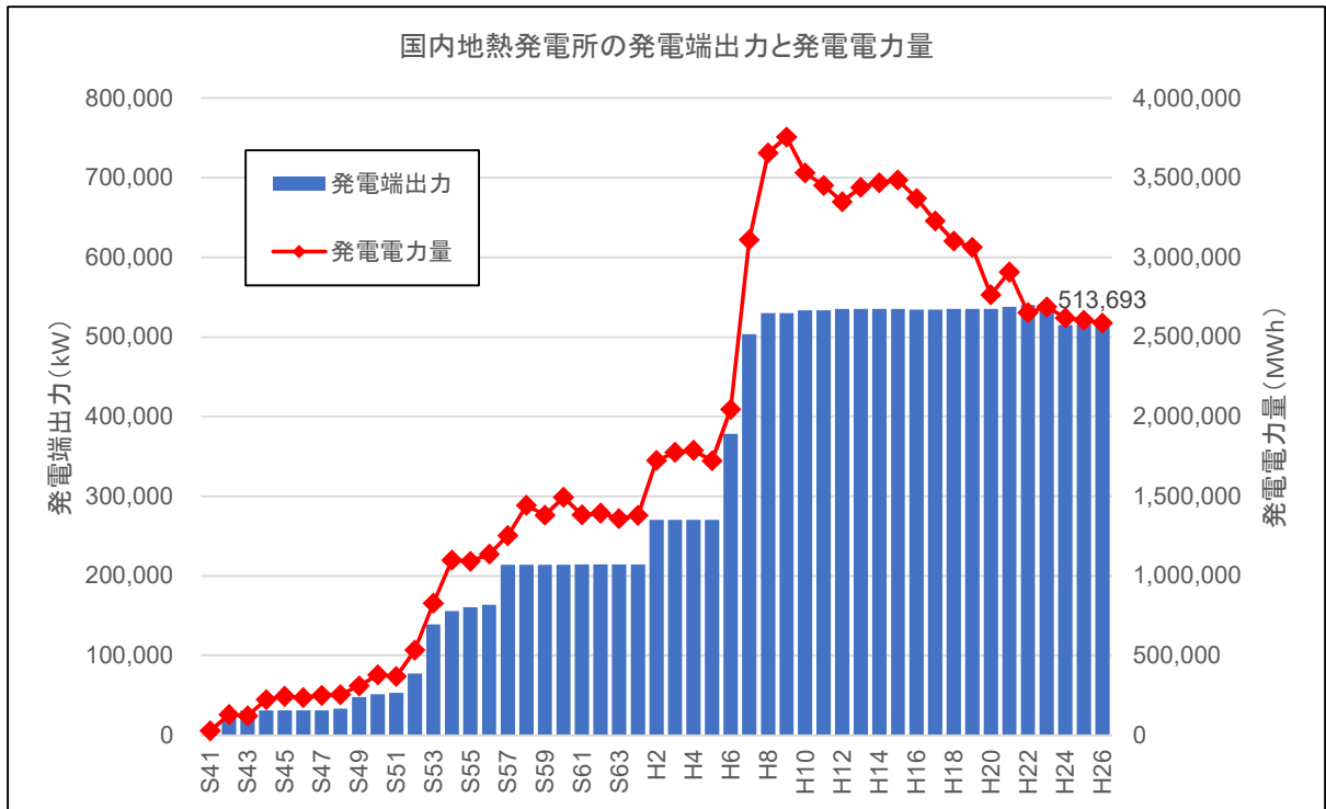
図4 国内地熱発電所の発電端出力と発電電力量の推移 火力原子力発電技術協会 (2015) 地熱発電の現状と動向より引用
