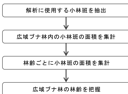
図 3-5 広域ブナ林の林齢の解析フロー
