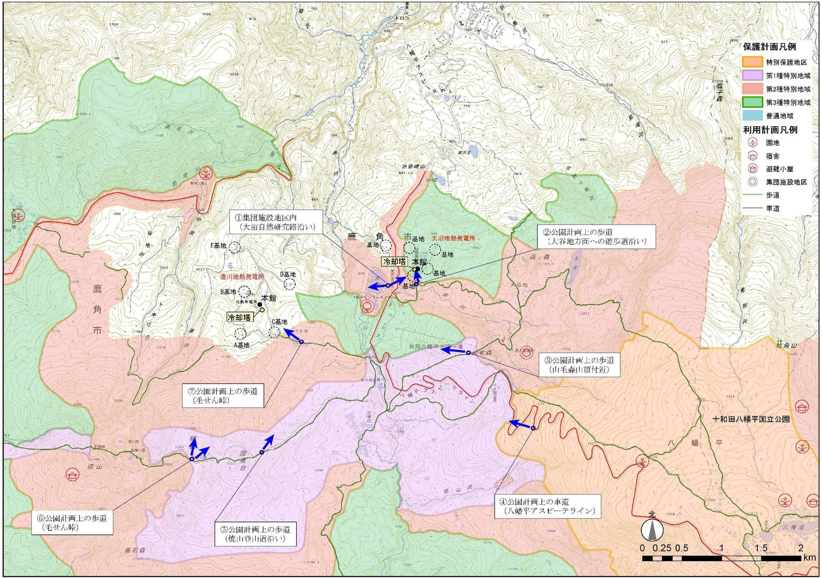
図1. 澄川、大沼地熱発電所・景観補足調査地点
