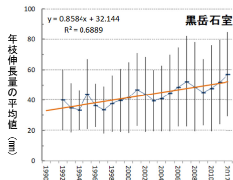
図 II-27 大雪山サイト黒岳石室のヒノキの年 枝伸長量
