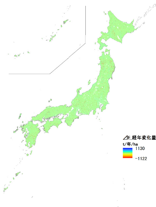
図 III-35 年間土壌流失防止量 (1983-1986 年度～1994-1998 年度)
