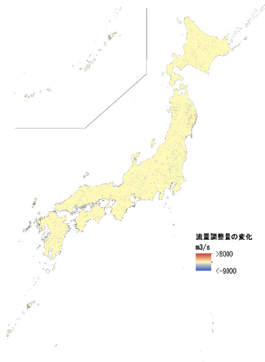
図 III-36 ピーク流量調整量の変化 (1983-1986 年度～1994-1998 年度)
