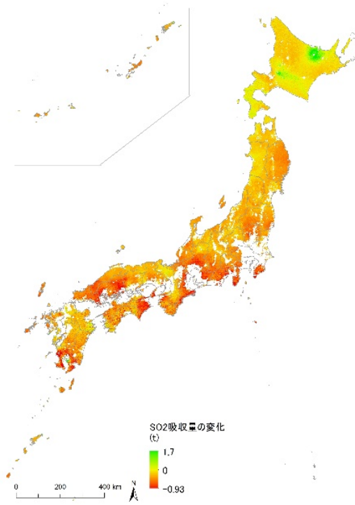
図 III-28 \text{SO}_2 吸収量の変化 (2000年と2010年の比較)
