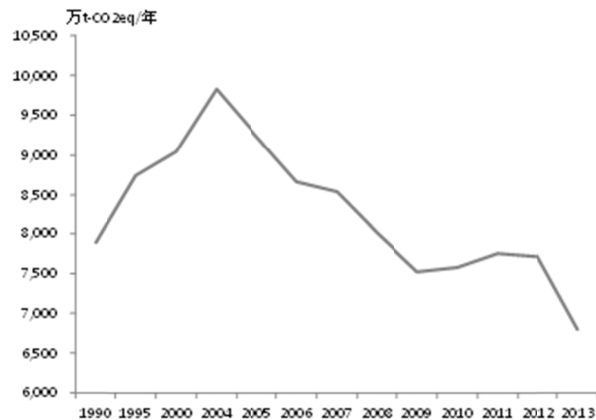
図 III-29 森林による炭素吸収量の推移
