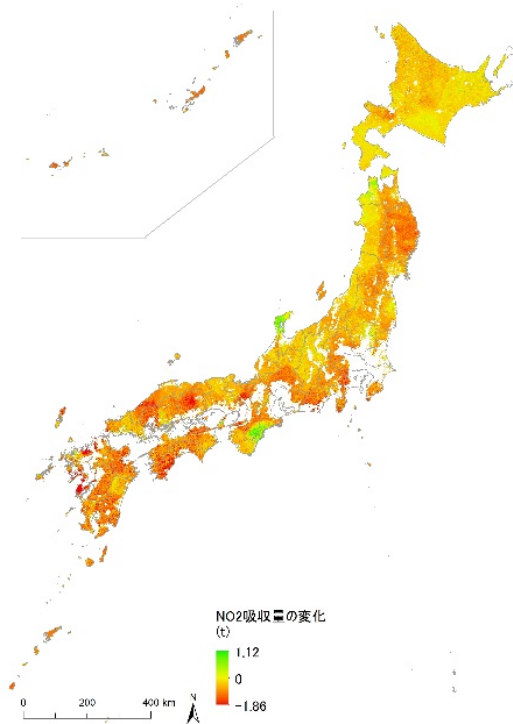
図 III-27 \text{NO}_2 吸収量の変化 (2000年と2010年の比較)
