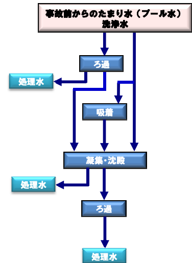
<水処理フローの例>
