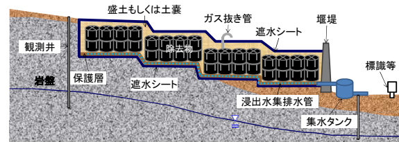
斜面を利用した設置例
