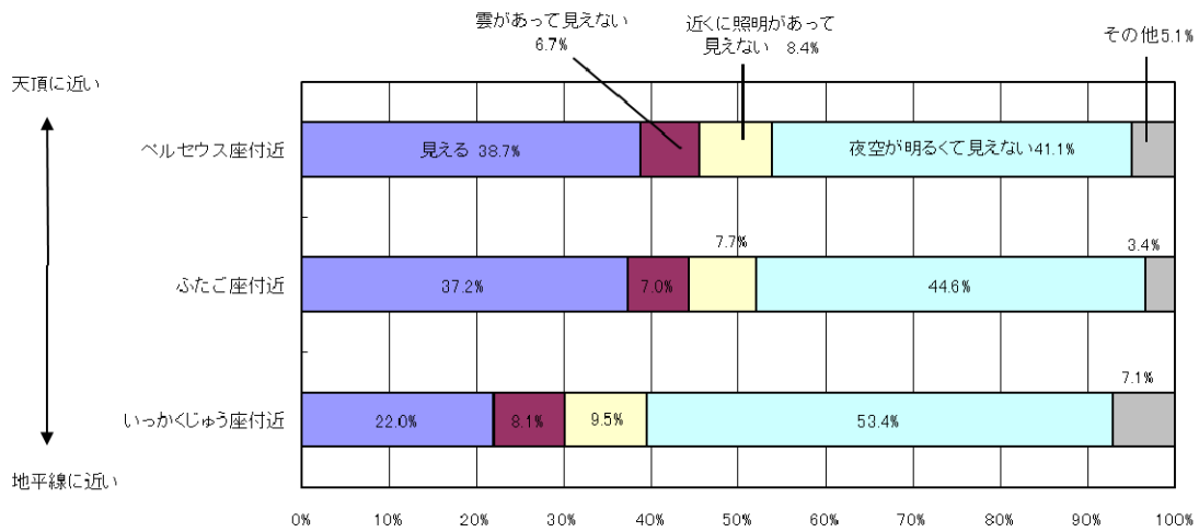
図3 肉眼による天の川の観察(冬期)
