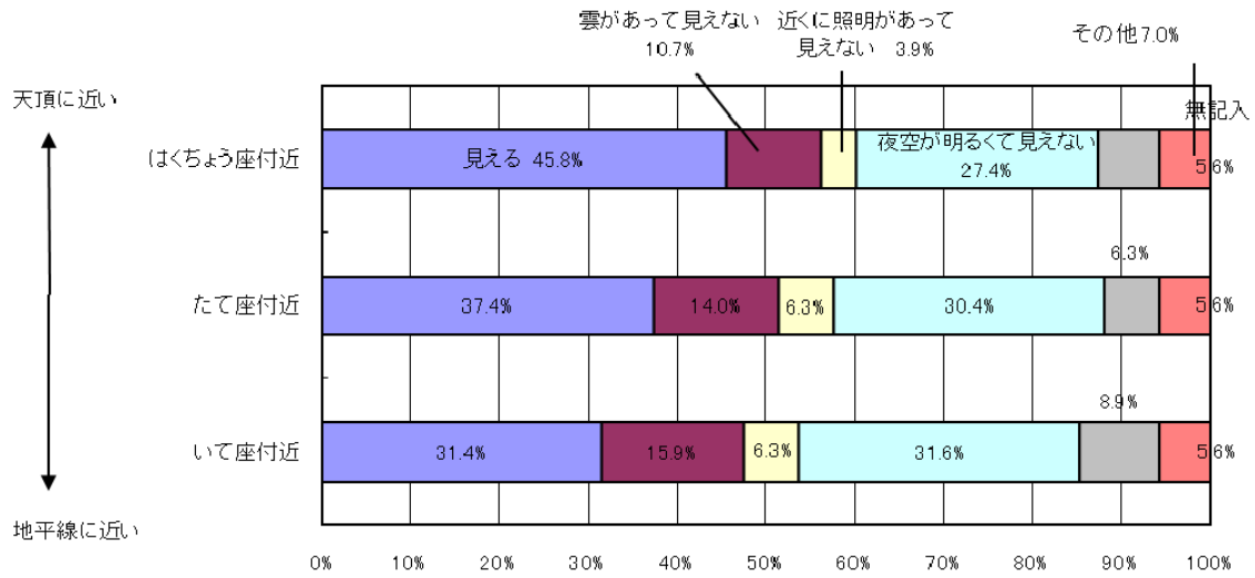
図2 肉眼による天の川の観察(夏期)
