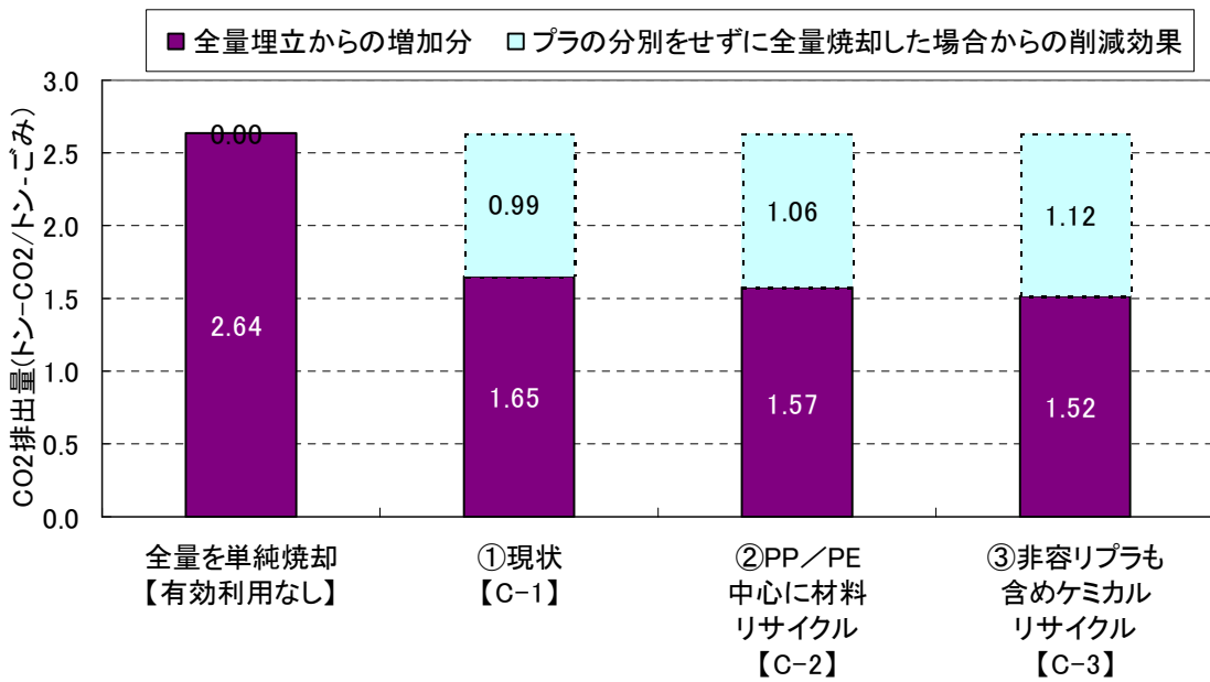
図 21 検討テーマ C における環境負荷とその削減効果 (CO2 排出量、ごみ 1 トンあたり)
