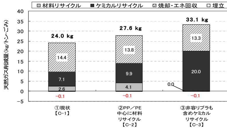
図 24 検討テーマ C における環境負荷削減効果の内訳 (天然ガス、ごみ 1 トンあたり)
