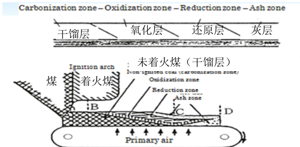
图 2.4-1 顺送链式炉炉箄子的燃烧机构
