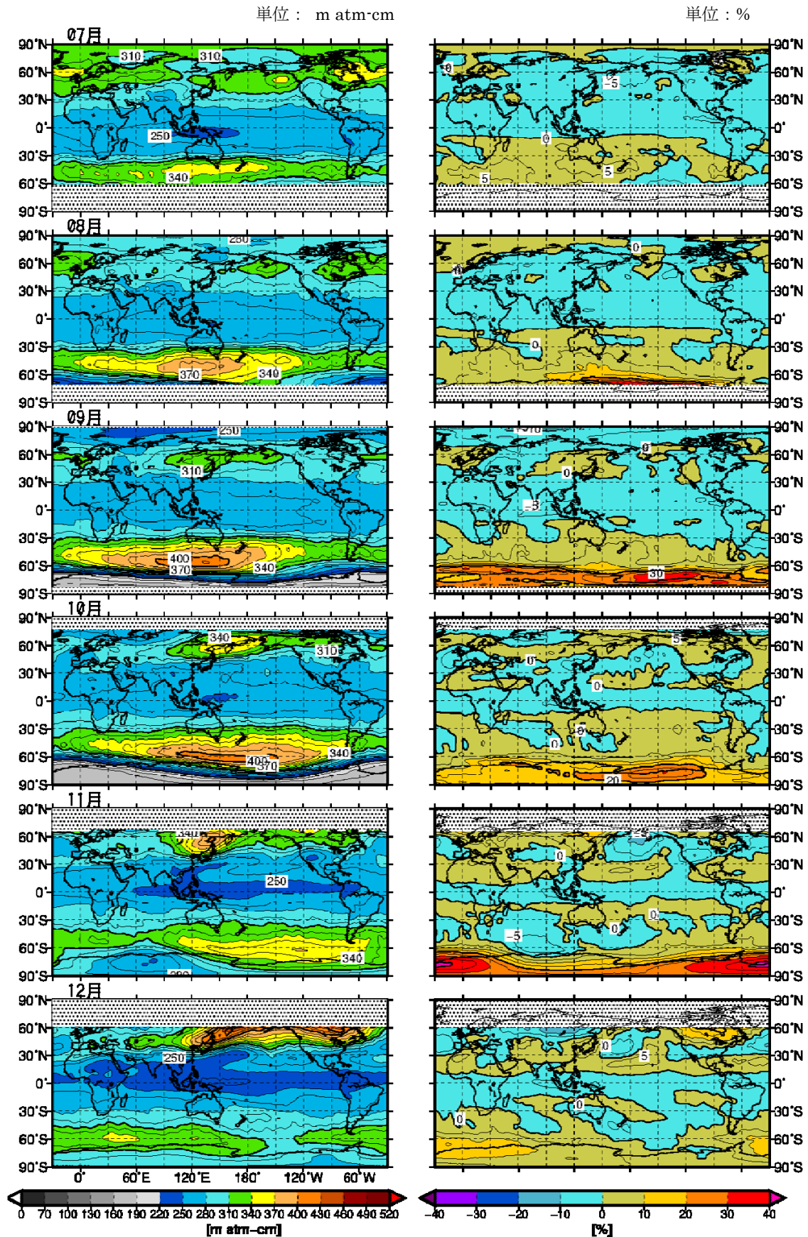
図1-資-2 月平均オゾン全量・偏差(%)の地球規模の分布図(2017年7~12月)
