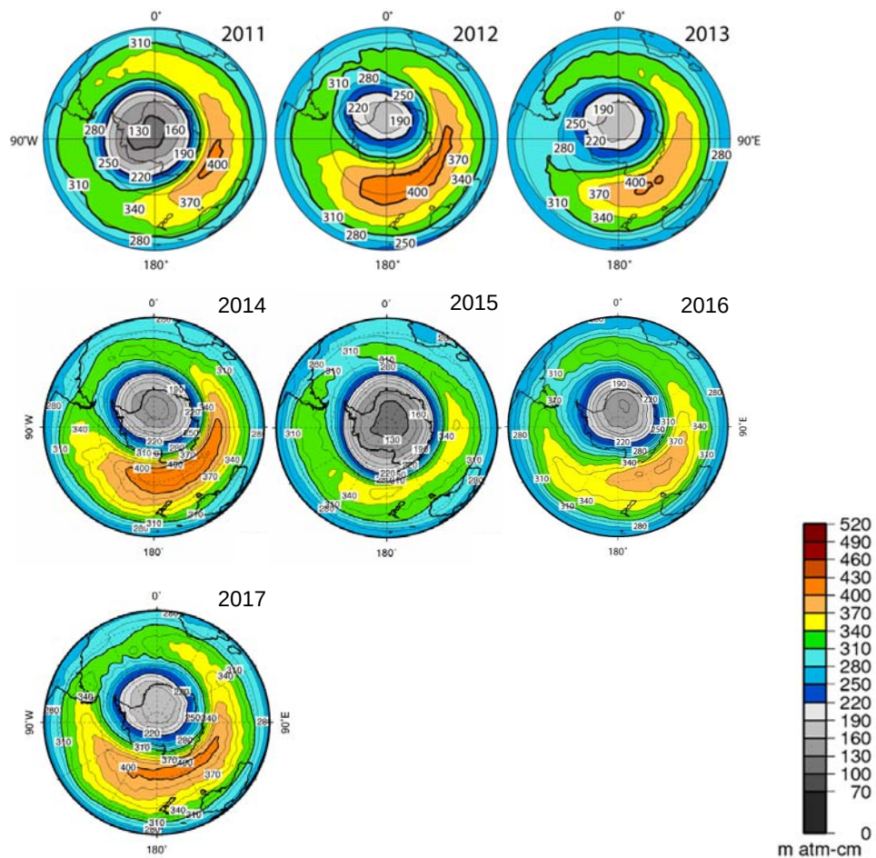
図1-資-5 10月の南半球月平均オゾン全量分布図（2011～2017年） （出典）気象庁提供データ
