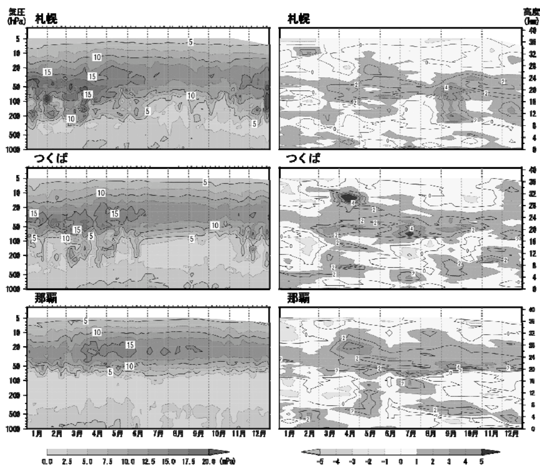
図1-資-7 国内3地点のオゾン分圧(左)と規格化偏差(右)の高度分布(2017年) 上から札幌、つくば、那覇のオゾンゾンデ観測によるオゾン分圧・偏差の高度分布図。オゾン分圧図(左)は個々の観測値を用い、規格化偏差図(右)は月平均値から作成。
