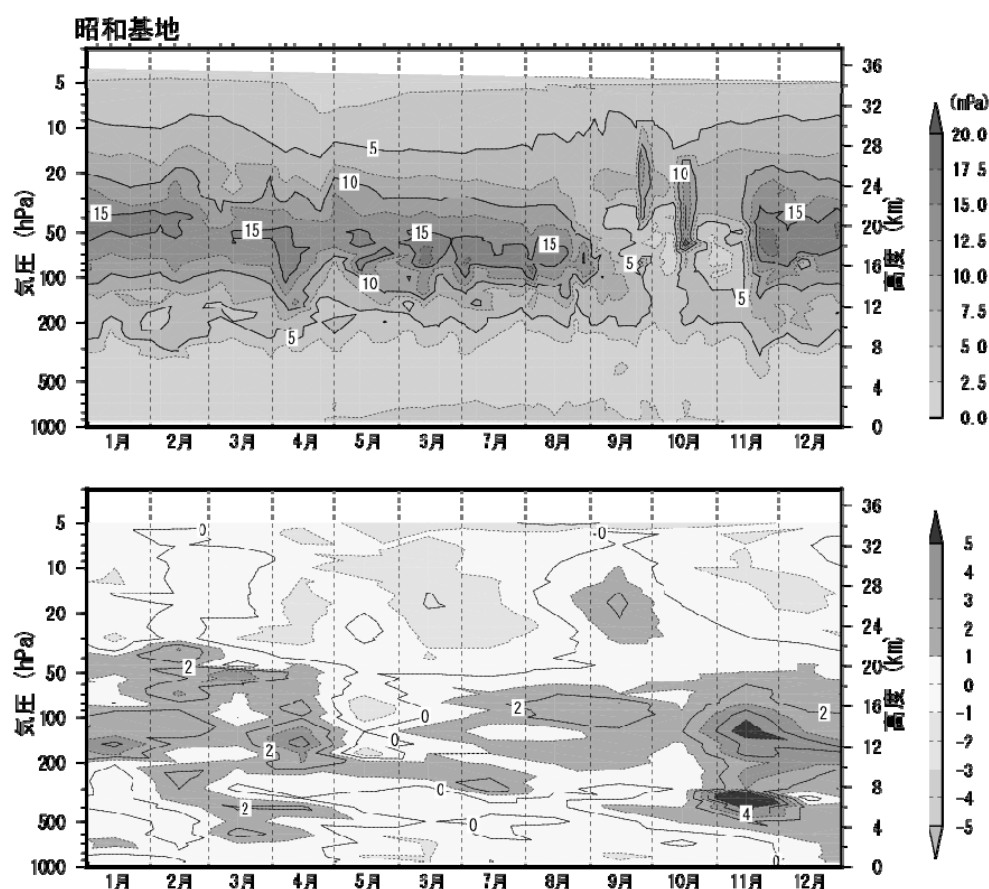
図1-資-8 南極昭和基地のオゾン分圧（上）と規格化偏差（下）の高度分布（2017年）
