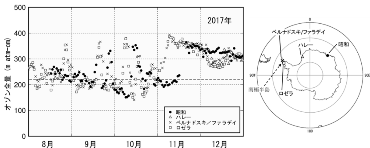
図1-資-6 南極域各国基地におけるオゾン全量の変化（2017年）
