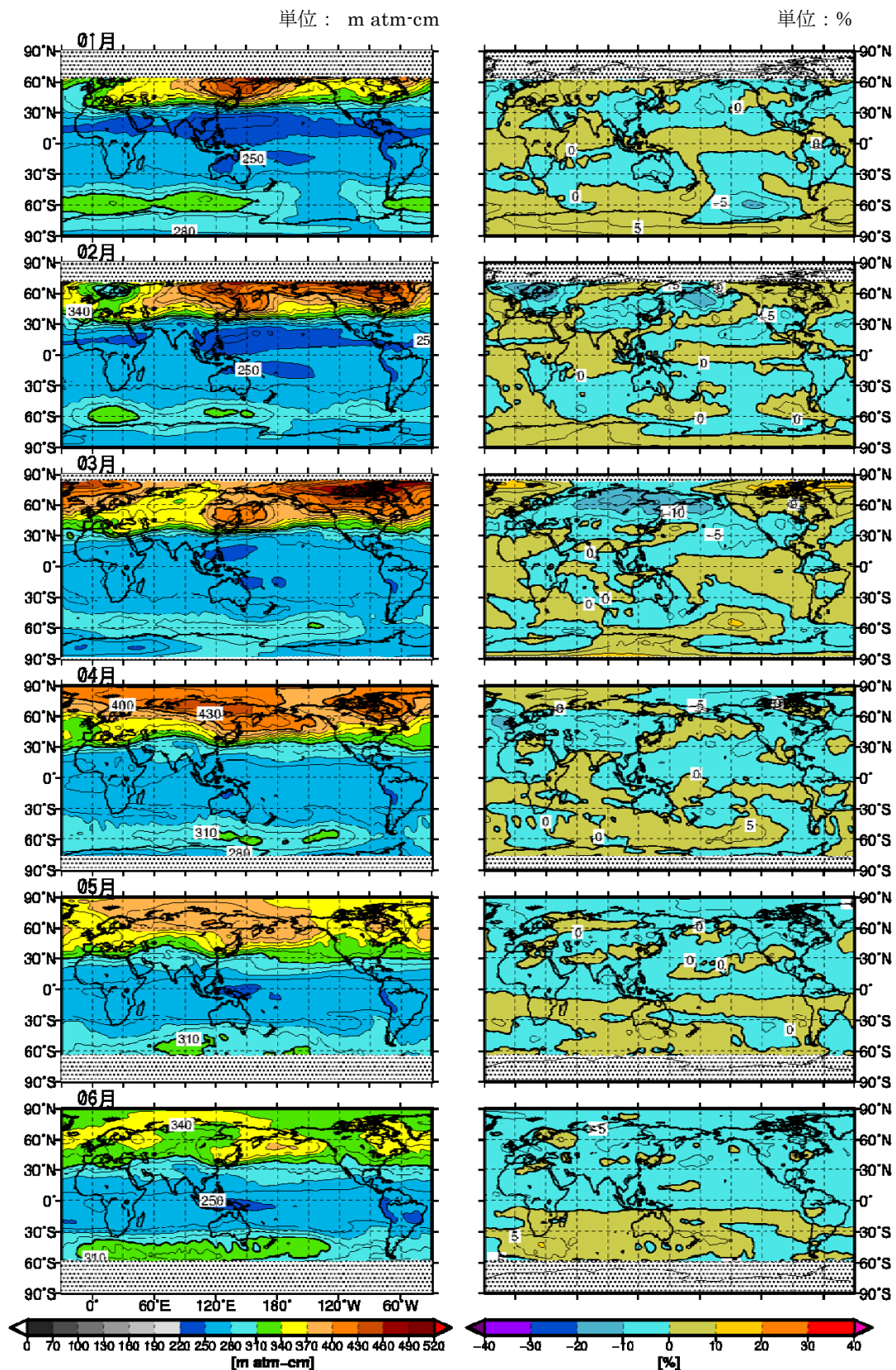
図1-資-1 月平均オゾン全量・偏差(%)の地球規模の分布図(2017年1~6月) (出典) 気象庁 オゾン層・紫外線の年のまとめ(2017年)より
