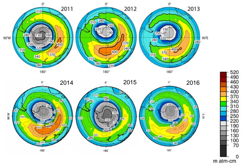
図1-資-5 10月の南半球月平均オゾン全量分布図（2011～2016年） （出典）気象庁提供データ
