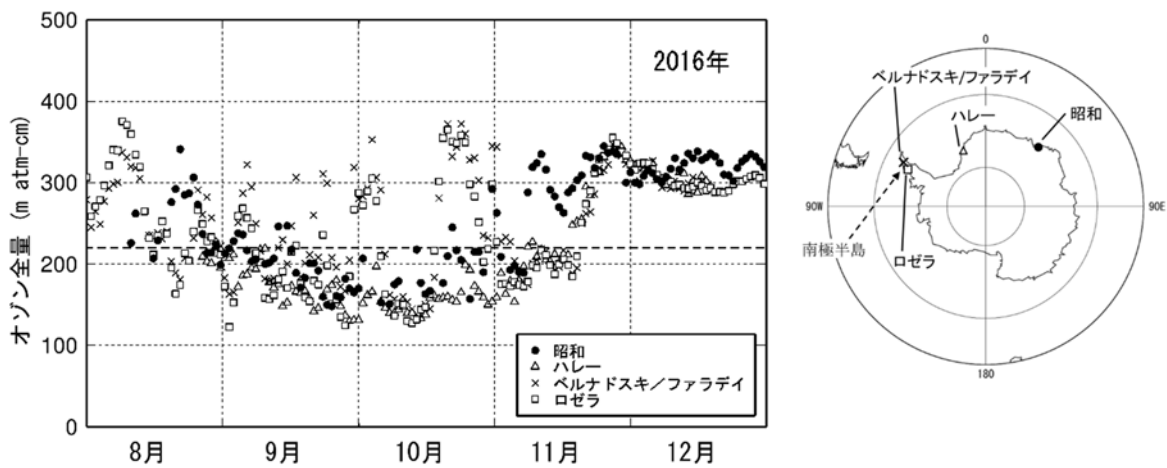
図1-資-6 南極域各国基地におけるオゾン全量の変化（2016年） （出典）気象庁 オゾン層・紫外線の年のまとめ（2016年）より
