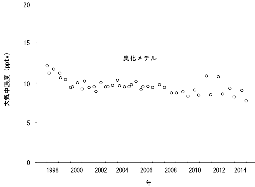
図 2-3-7 北海道における臭化メチルの大気中のバックグラウンド濃度の経年変化 (出典) 環境省 平成 26 年度フロン等オゾン層影響微量ガス等監視調査より
