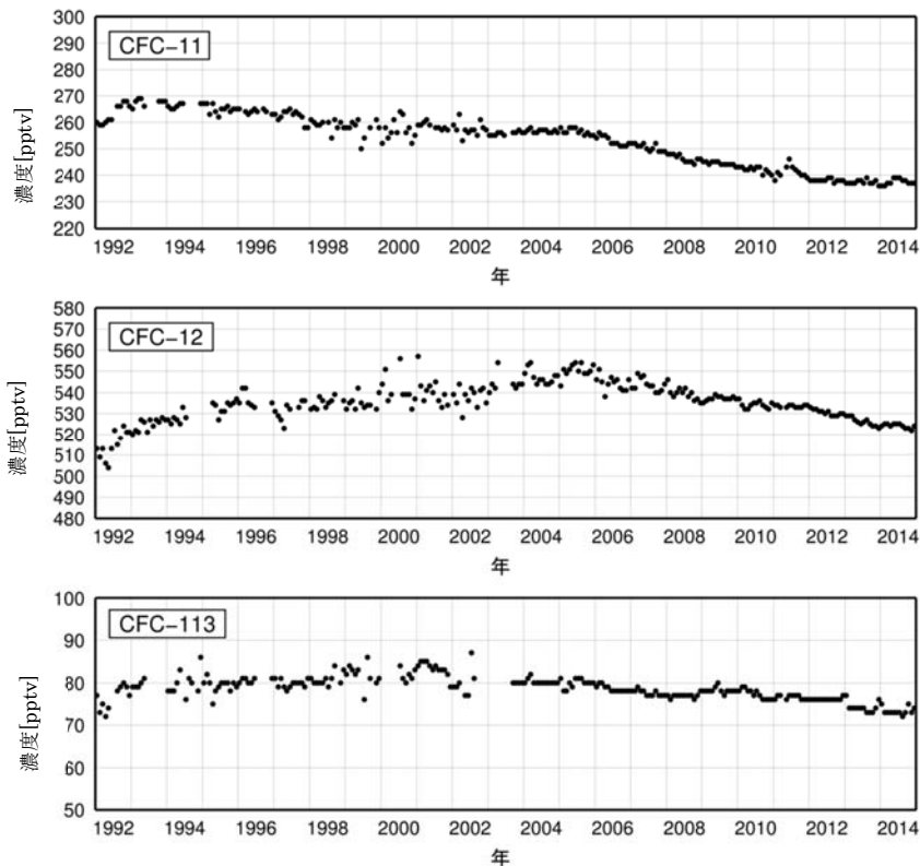
図 2-3-9 岩手県大船渡市綾里における大気中のクロロフルオロカーボン類濃度の経年変化 綾里における大気中の CFC-11（上）、CFC-12（中）、CFC-113（下）の地上での月平均濃度（測定結果を月平均したもの）の経年変化を示す。なお、データの無い期間は、主に観測機器の更新や校正作業のための欠測である。また、観測精度を向上させるため、2003 年 9 月から放射線源を用いた電子捕獲型検出器（ECD）を搭載したガスクロマトグラフを導入したことにより、観測濃度データのばらつきがそれ以前と比較して少なくなっている。※口絵 IV 参照。口絵では、水色で表している。
