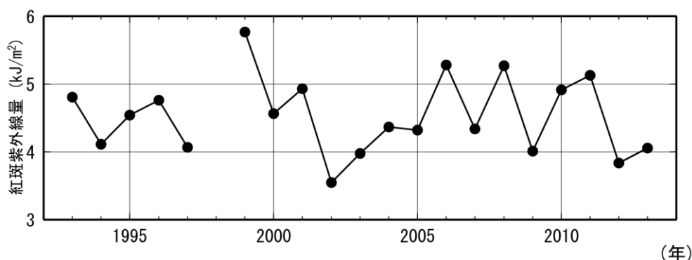
図 3-3-5 1993 年から 2013 年までの南極昭和基地における 11～1 月平均紅斑紫外線量日積算値の経年変化
