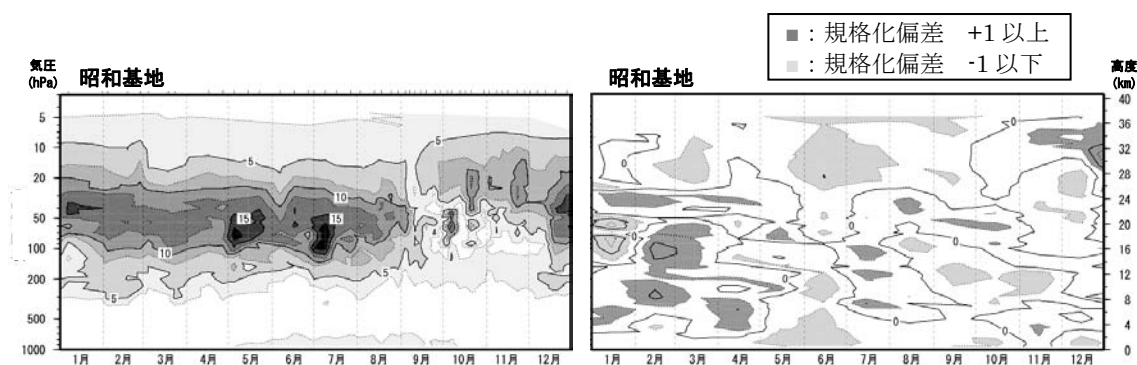
図1-資-8 南極昭和基地のオゾン分圧(左)と規格化偏差(右)の高度分布(2011年) 南極昭和基地のオゾンゾンデ観測によるオゾン分圧・規格化偏差図。オゾン分圧図(左)は個々の観測値を用い、規格化偏差図(右)は月平均値から作成。規格化偏差は月平均値の参照値からの偏差を標準偏差で割った値。なお、観測データのない高度については、前後の期間のオゾン分圧から内挿処理を行っている。(出典) 気象庁 オゾン層・紫外線の年のまとめ(2011年)
