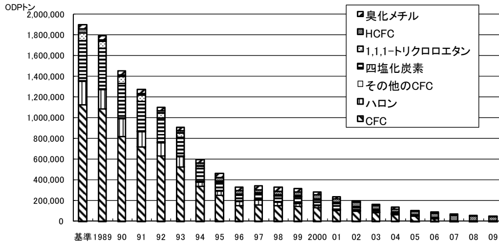
図 4-2 モントリオール議定書に基づくオゾン層破壊物質の生産量の推移 (1989～2009年) ただし、基準年以前の空白データは基準年で一定として補完 (HCFC を除く) し、基準年と規制開始の間の空白データは一定の割合で変化するものとして補完 (先進国の HCFC については 1990 年・1991 年のデータを補完)。単位は ODP トン。 (出典) UNEP オゾン事務局ウェブサイト
