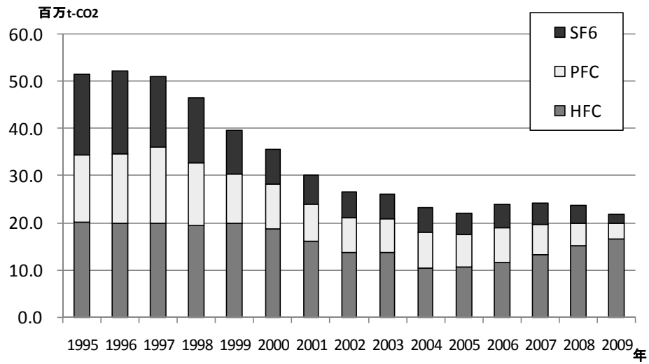
図 4-12 代替フロン等 3 ガスの排出量の推移 (ガス別)
