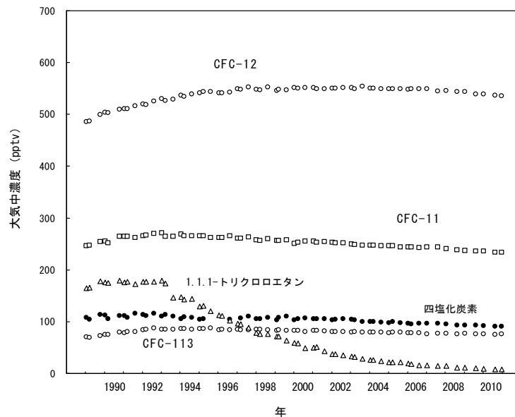
図 2-3-1 北海道における特定物質の大気中のバックグラウンド濃度の経年変化 ※口絵 IV 参照。口絵では、紫色で表している。 (出典) 環境省 平成 22 年度フロン等オゾン層影響微量ガス等監視調査
