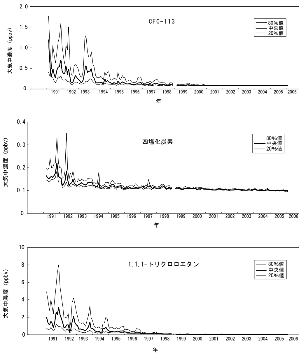
図 2-3-15 川崎市における特定物質等の月別濃度（中央値）の経年変化（続き） （出典）環境省 平成 17 年度フロン等オゾン層影響微量ガス等監視調査 及び平成 22 年度フロン等オゾン層影響微量ガス等監視調査
