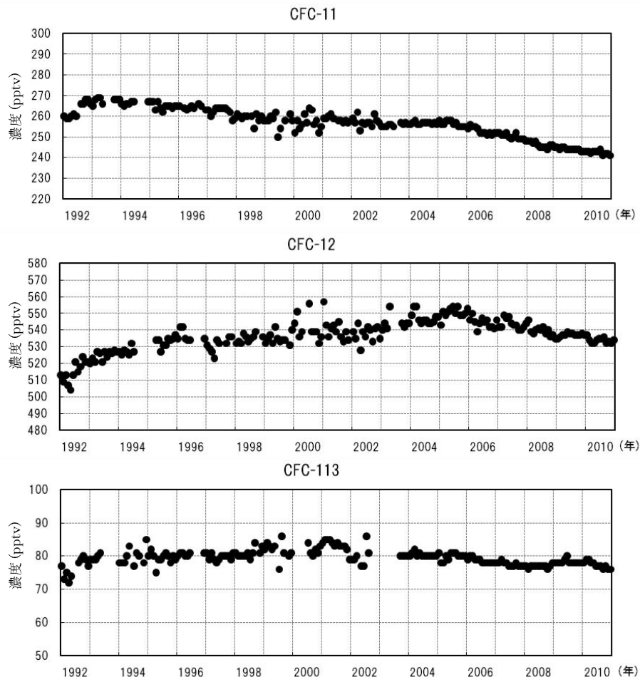
図 2-3-8 岩手県大船渡市綾里における大気中のクロロフルオロカーボン類濃度の経年変化
