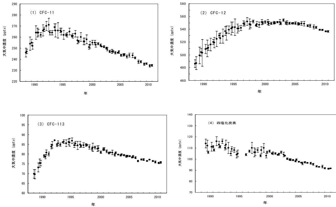
図 2-3-2 北海道における CFC-11、CFC-12、CFC-113 及び四塩化炭素の大気中のバックグラウンド濃度の経年変化
