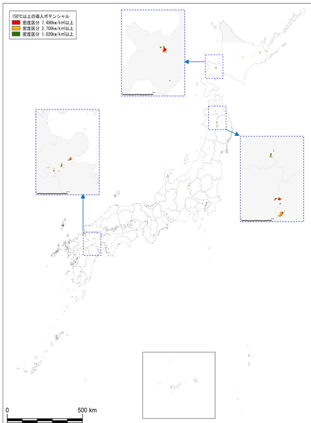
図5 地熱発電の導入ポテンシャル分布(150°C以上)
