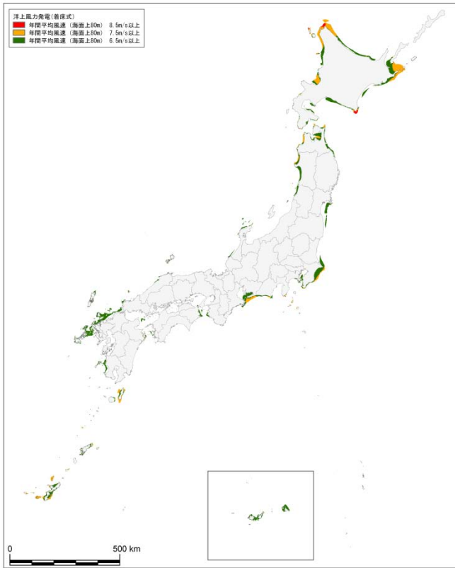
図2 洋上風力発電(着床式)の導入ポテンシャル分布
