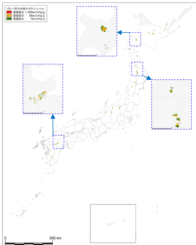
図 6 地熱発電の導入ポテンシャル分布(120～150℃)
