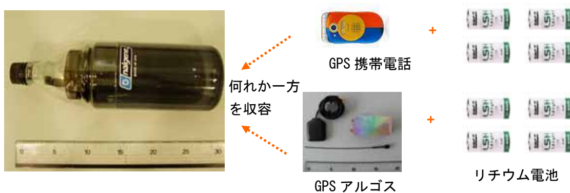
図 5.1-1 調査に用いた発信機と容器
