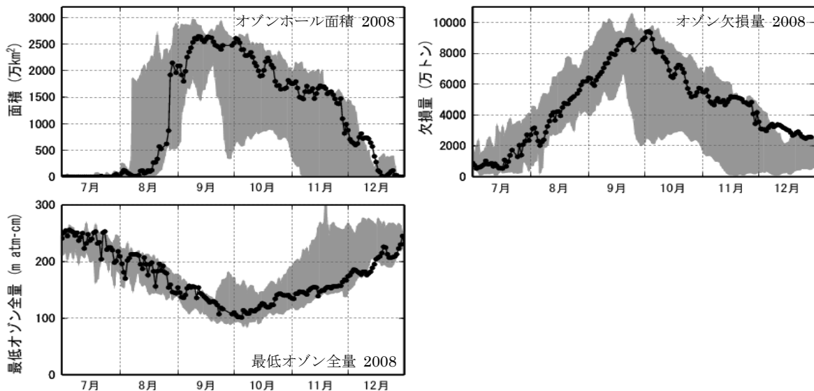
図 1-3-14 オゾンホール規模の推移 (2008 年 7 月～2008 年 12 月)
