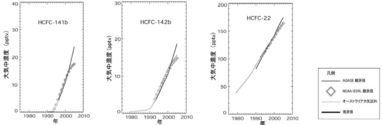
図 2-3-12 海外のネットワークで観測された HCFC-22、HCFC-141b 及び HCFC-142b の濃度変動 「オーストラリア大気試料」は、モデルを用いて全球平均値を算出している。推測値は、Scientific Assessment of Ozone Depletion:2002 (WMO, 2003) における Ab シナリオ (モンテリオール議定書北京改正 (1999 年) に定められた生産量・消費量規制が遵守されると想定したシナリオ) に基づく 1990 年代初頭から 2005 年までのもの。計算に用いた半減期は、それぞれ 9.3、17.9、12.0 年。 (出典) Scientific Assessment of Ozone Depletion:2006 (WMO, 2007)
