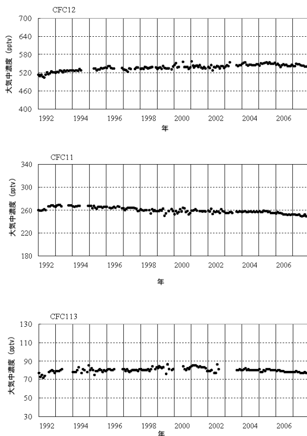
図 2-3-7 岩手県大船渡市綾里における大気中のクロロフルオロカーボン類濃度の経年変化 綾里における大気中の CFC-12 (上)、CFC-11 (中)、CFC-113 (下) の月平均濃度の経年変化を示す。 (出典) 気象庁 オゾン層観測報告:2007
