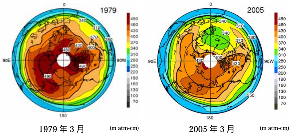
図 1979年及び2005年における3月の月平均オゾン全量の北半球分布 出典：気象庁提供データ
