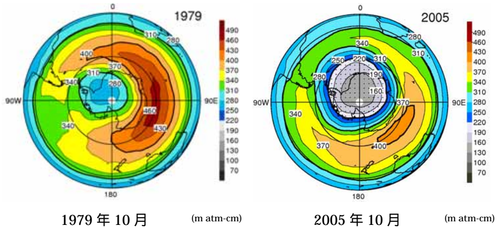
図 1979年及び2005年における10月の月平均オゾン全量の南半球分布 p.28～30 図17として掲載 出典：気象庁提供データ
