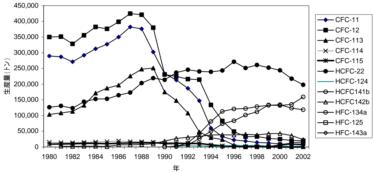
図 71 主要なフロンの年別生産量の推移 (1980~2002年)
