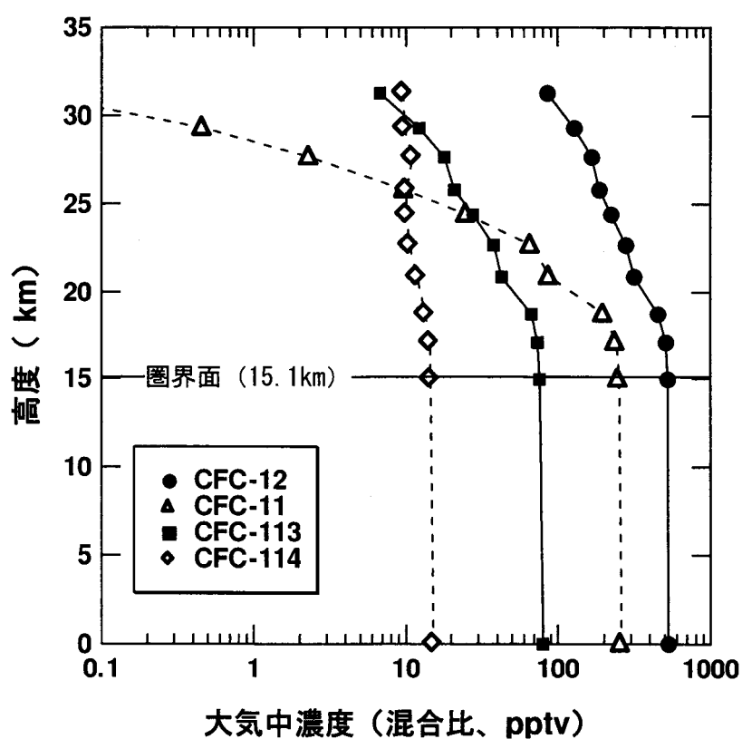
図 44 三陸上空におけるCFC-11、CFC-12、CFC-113、CFC-114の高度分布 (2000年8月28日)
