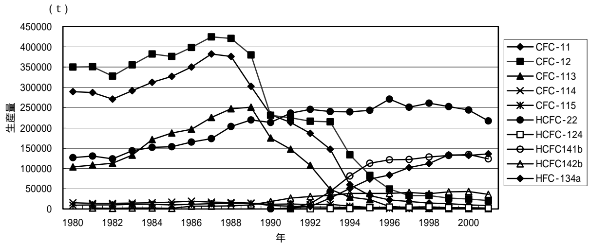
図 58 主要なフロンの年別生産量の推移 (1980 ~ 2001 年)
