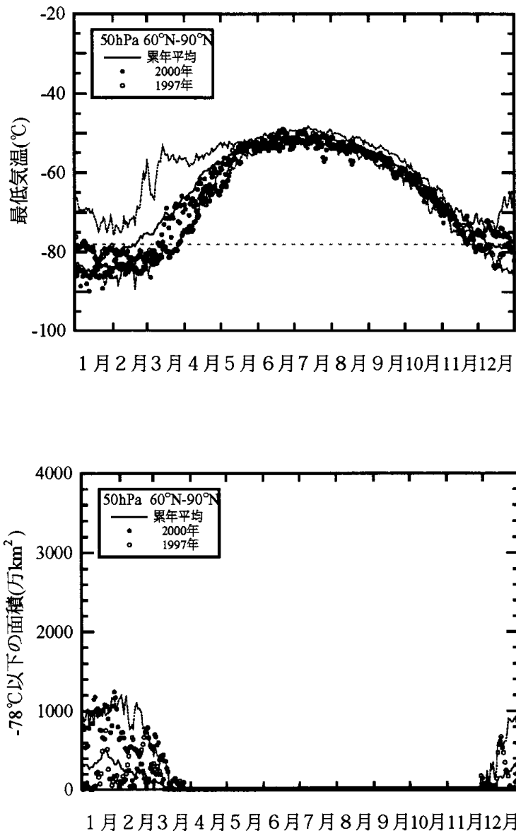
図 28 北緯 60 度以北における 50hPa の最低気温、及び気温が - 78 以下の領域の面積の推移 ( 2000 年 1 ~ 12 月 )
