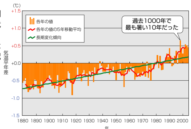
■ 世界の年平均地上気温の年差（陸上のみ）（1880～2004年）
