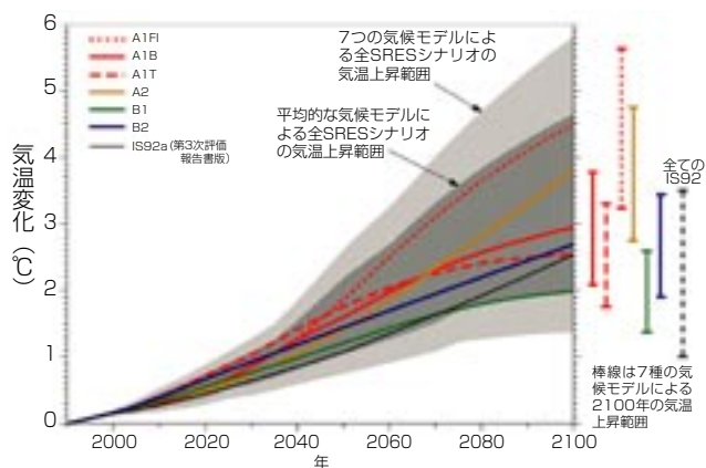
■ SRESシナリオによる気温上昇の予測 (文献15より)
