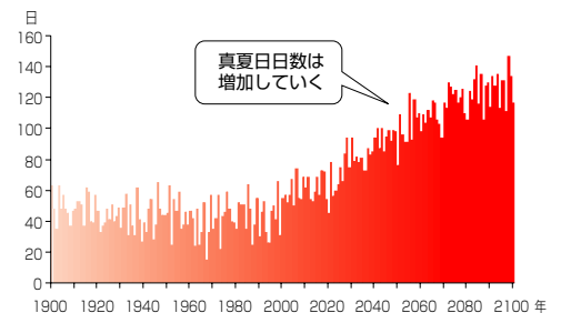
■ 日本の真夏日日数の変化 (1900～2100年)
