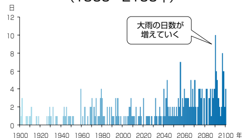
■ 日本の夏季 (6, 7, 8月) の大雨日数の変化 (1900～2100年)
