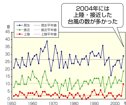
■ 台風の発生、接近、上陸個数 （文献8より）
