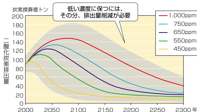
■ 様々な安定化水準に対応する世界の二酸化炭素排出量の変化（文献24より）
