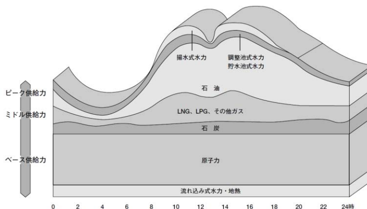
図表 2 現状の電源構成
