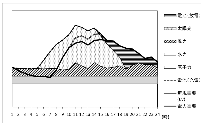
図表 3 ゼロカーボン電源による需給のイメージ
