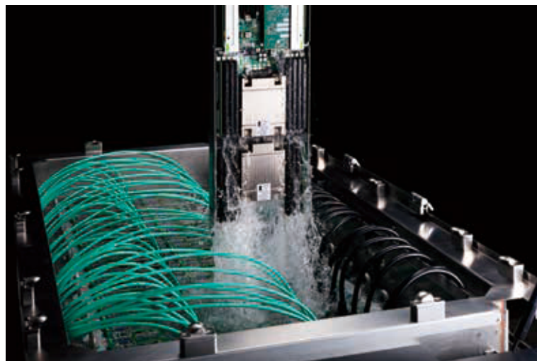
液浸冷却システムによるCO 2 排出削減
