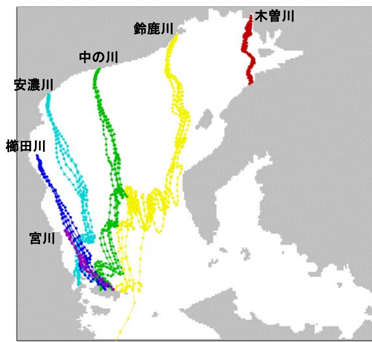
図 9 アルゴスポトルの漂流経路
