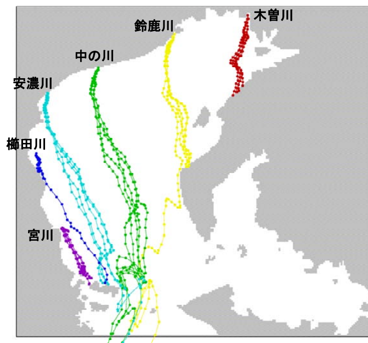
図 10 携帯ボトルの漂流経路
