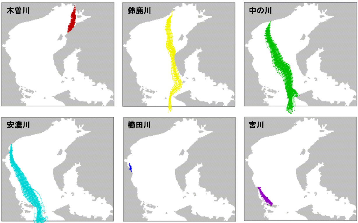
図 11 生分解性ボトルの漂流経路
