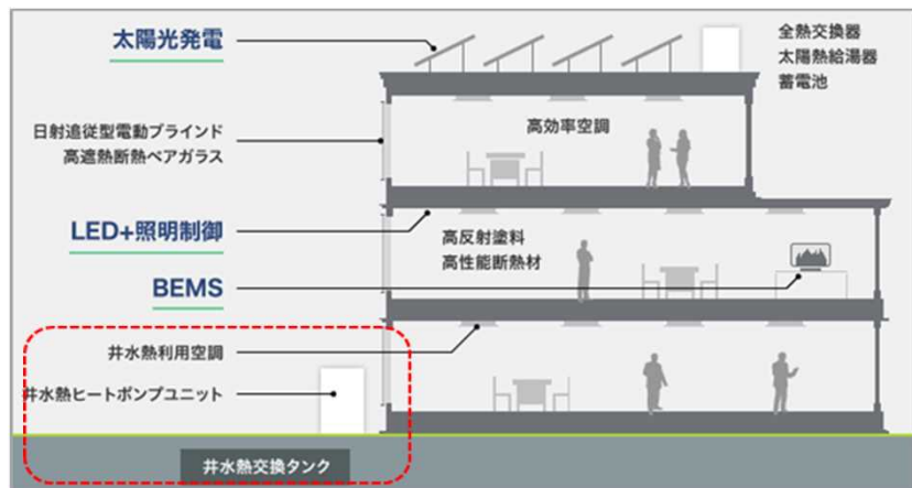
豊富な地下水を活用した井水熱利用空調システム
